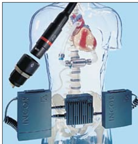
Рис. 7. Кардиологическая система
