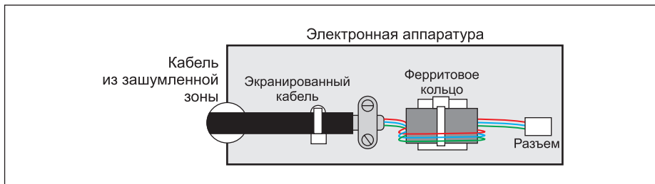
Рис. 4. Установка фильтра на основе ферритового кольца на контрольном кабеле, входящем в электронную аппаратуру
