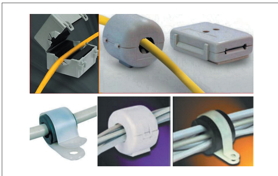
Рис. 3. Конструкция ферритовых фильтров для быстрого и удобного монтажа на проводах
