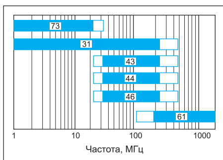
Рис. 5. Частотные диапазоны различных типов материалов (обозначены номерами), используемых в производстве ФЭ в компании Fire-Rite Products Corp.
