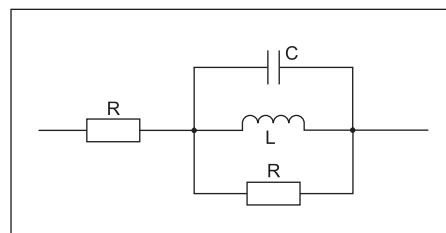
Рис. 7. Схема замещения фильтра на основе ФЭ
