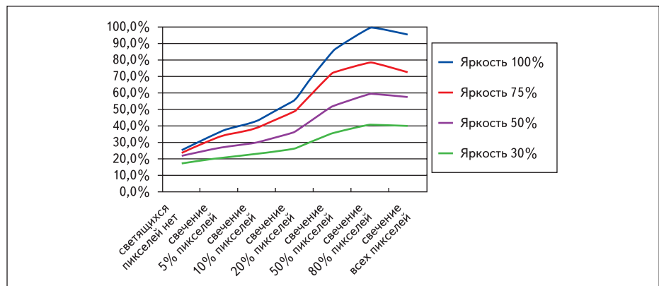
Рис. 9. Энергопотребление дисплея EL320.240.36-NB
