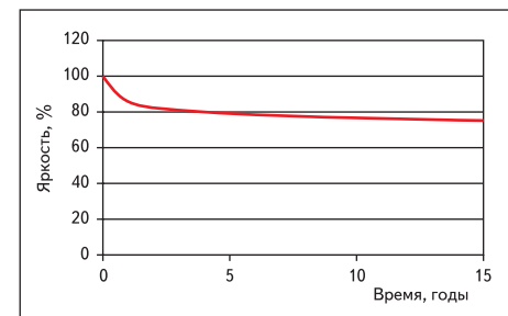
Рис. 4. Стабилизация яркости EL-дисплеев с течением времени
