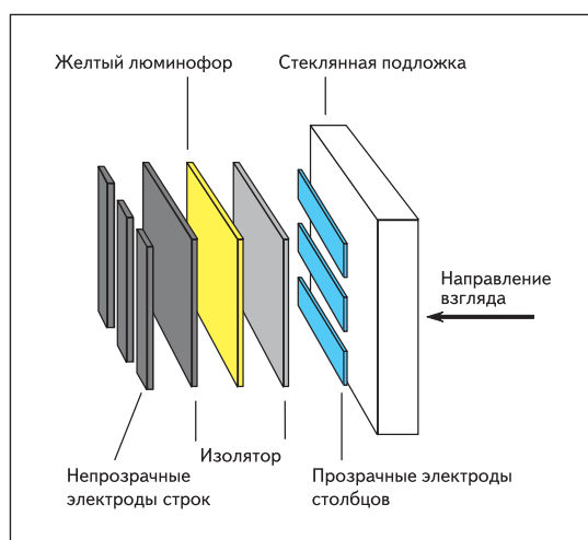
Рис. 2. Структура EL-дисплея
