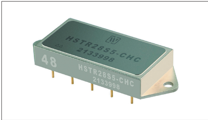
Рис. 11. Внешний вид DC/DC-преобразователя серии HSTR28 с монтажными фланцами
