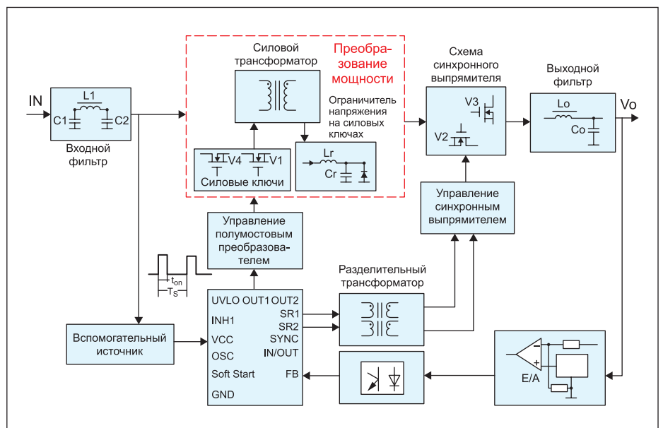
Рис. 13. Структурная схема одноканальной модели преобразователя серии HOL28 с синхронным выпрямителем
