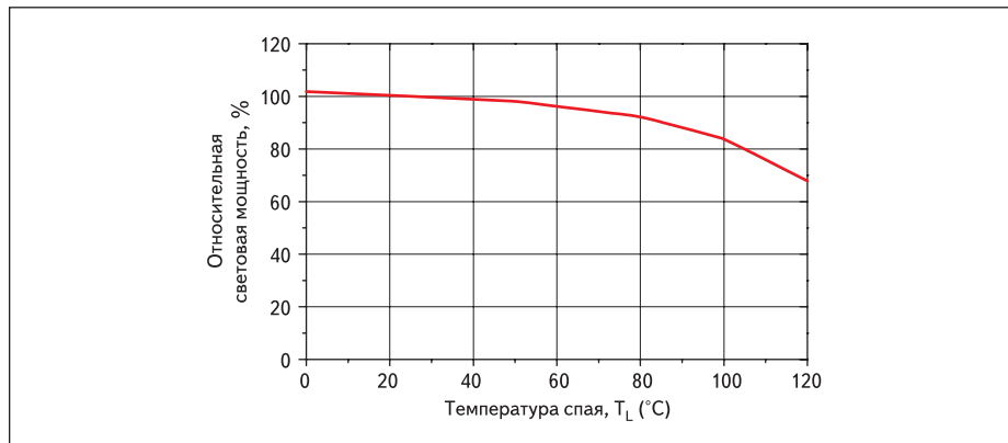
Рис. 2. Зависимость относительной световой мощности от температуры спая
