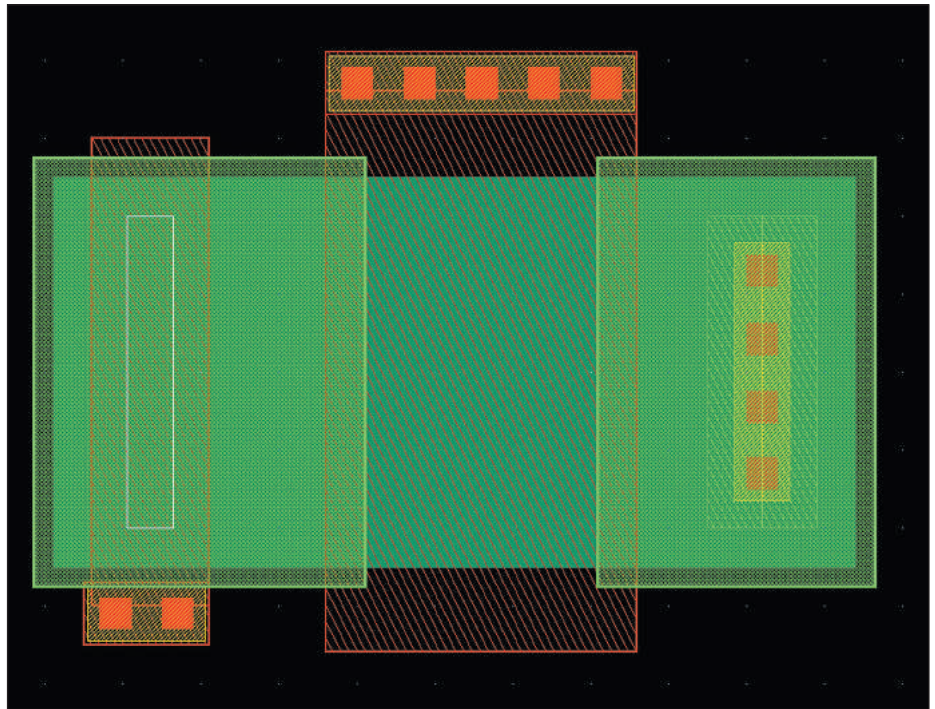
Рис. 2. Топология ячейки памяти микросхем 1645PT2U и 5576PT1U
