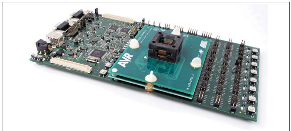
Рис. 2. Отладочная плата STK600
