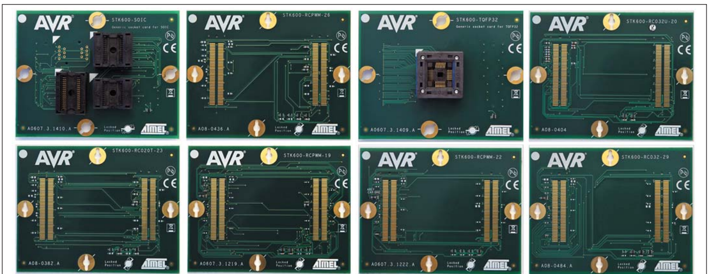
Рис. 3. Примеры наборов мезонинных плат для STK600
