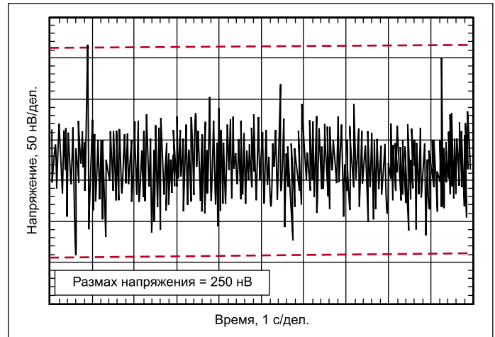
Рис. 1. Шум операционного усилителя OPAx188 в полосе частот от 0,1 до 10 Гц
