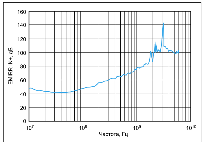
Рис. 2. Зависимость коэффициента ослабления электромагнитных помех (EMIRR IN+) от частоты для операционного усилителя OPAx188
